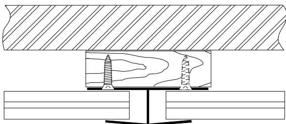
Anwendungsbeispiel! Mittelverbindung mit H-Profil - Art. Nr. 023 -
