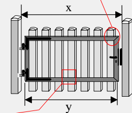
Pfostenabstand X ( Innenmaß ) - 80 mm = Rahmenmaß Y ( Außenmaß )
