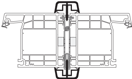
Anwendungsbeispiel Profine 76 mit Art. 450 / Art. 453
