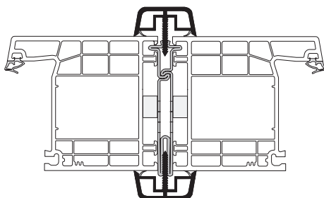
Anwendungsbeispiel Profile 76 mit Art. 450 / Art. 453
