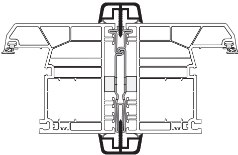
Anwendungsbeispiel Profine 88 mit Art. 450 / Art. 455
