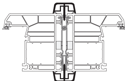
Anwendungsbeispiel Profile 88 mit Art. 450 / Art. 455
